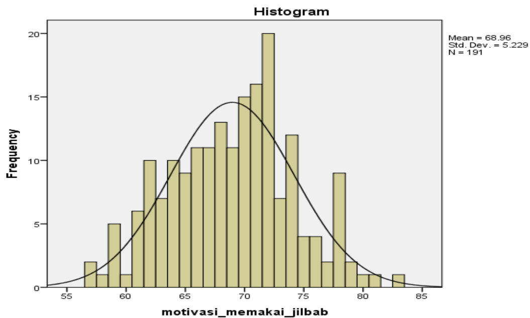
Gambar 4.1 Histogram Motivasi Memakai Jilbab
