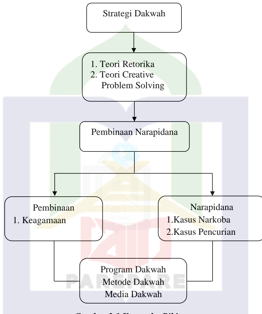
Gambar 2.1 Kerangka Pikir
