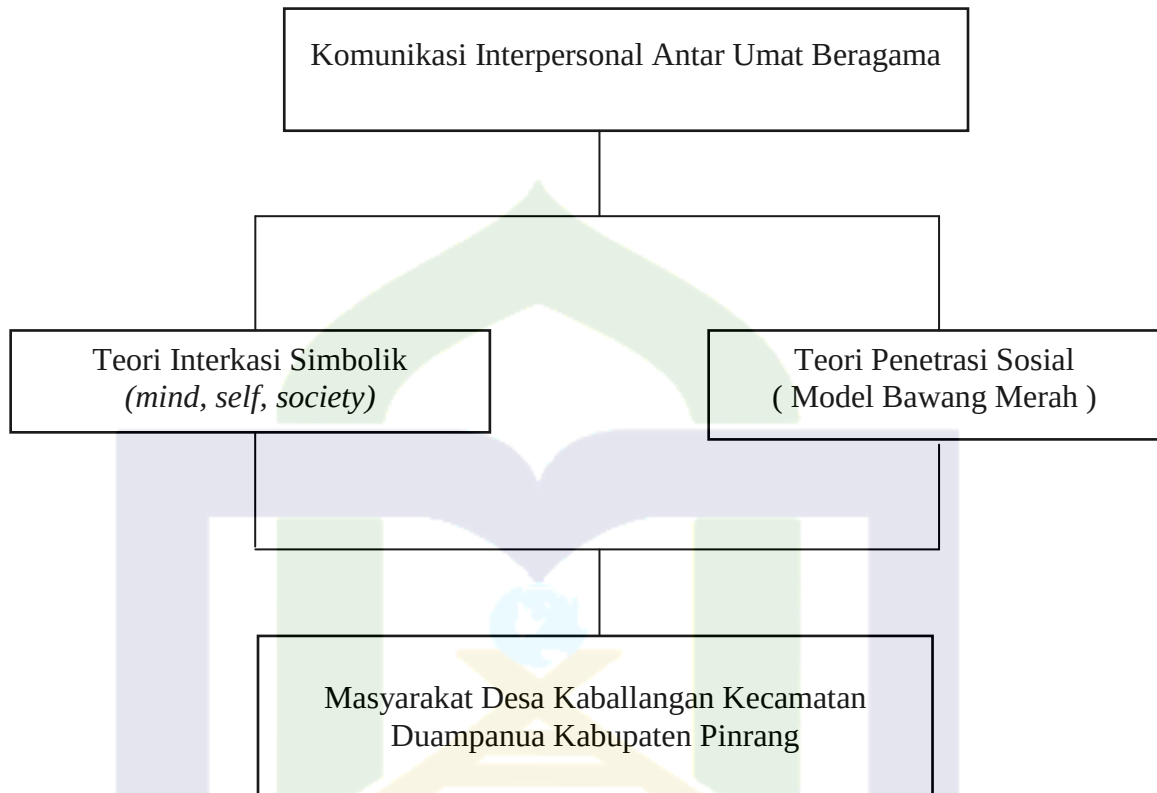
Gambar 1. Kerangka Pikir
