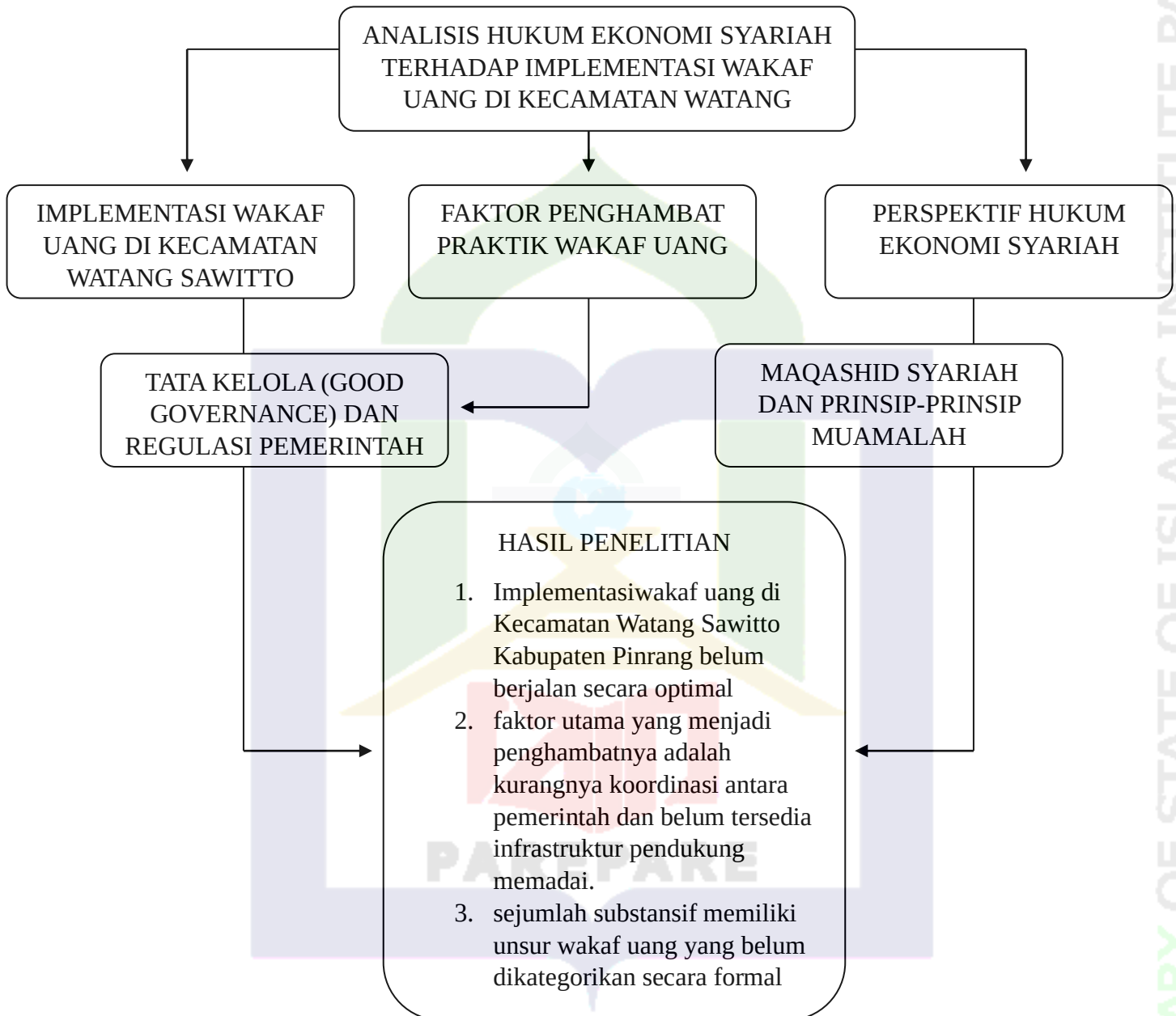
GAMBAR 1.1 KERANGKA PIKIR
