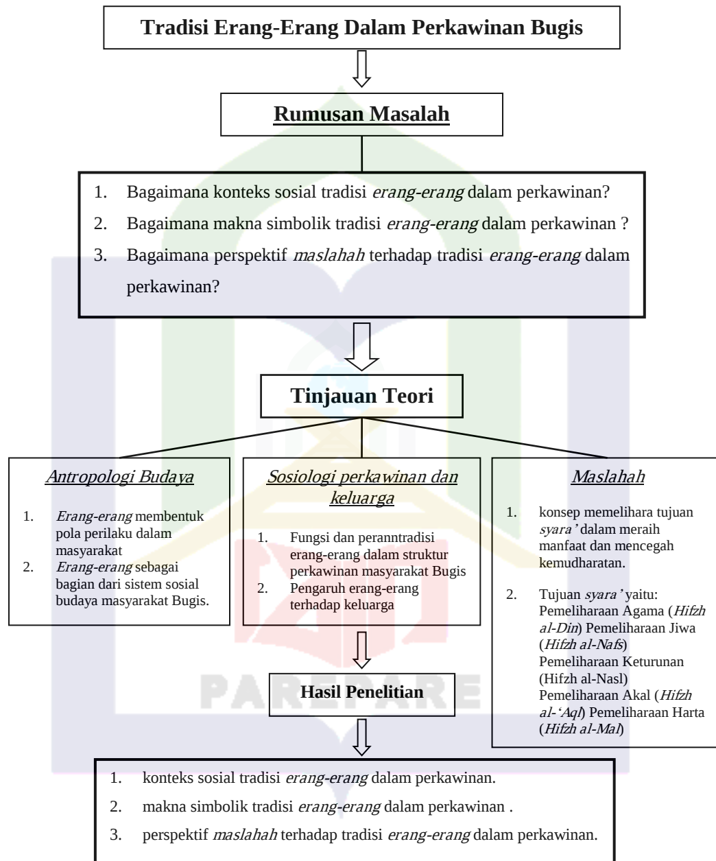
Gambar 1 Kerangka Pikir
